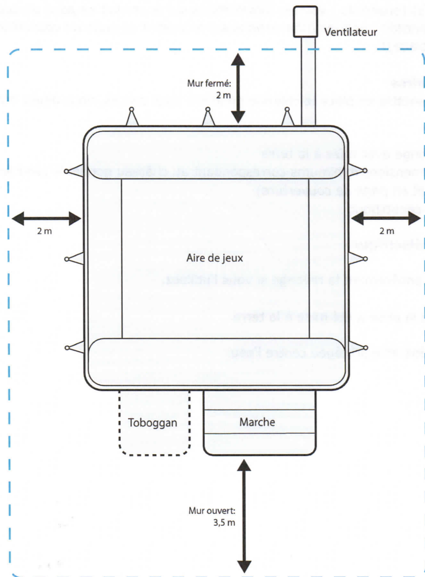
Figure 2 Espace libre minimum exigé autour du château gonflable (exemple de château gonflable général)
